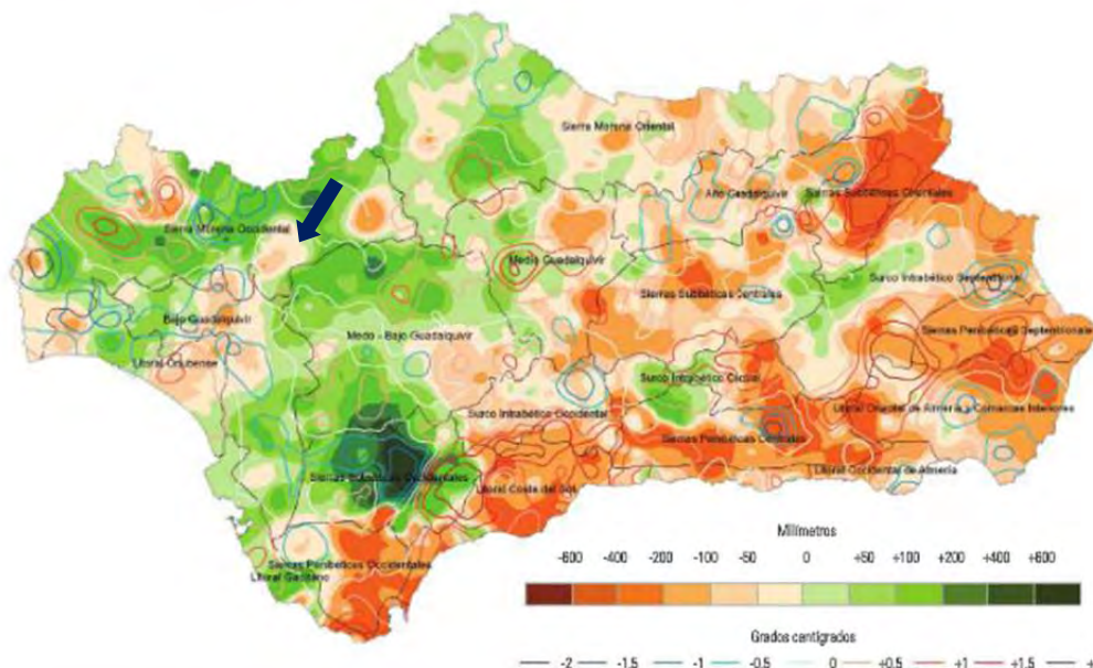
Mapa de desviaciones de las precipitaciones y temperaturas anuales de 2014 respecto a la media 1971-2000
